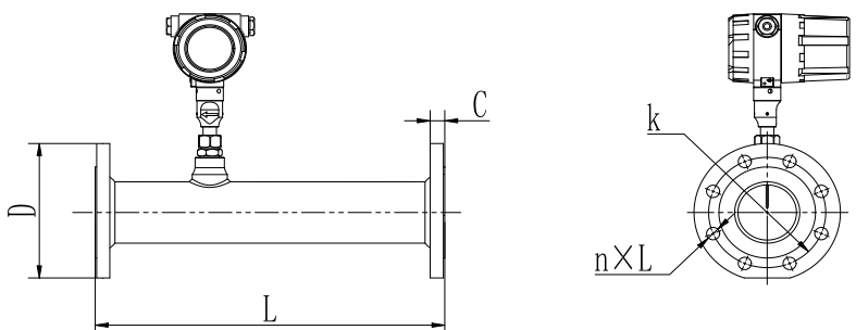
GB/T9119-2000 PN1.6Mpa (16bar) 平面、突面板式平焊钢制管法兰 (单位: mm)
