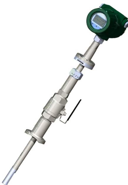
图 1 适用管径 DN100 以上 DN500 以下 精简型热式气体质量流量计
