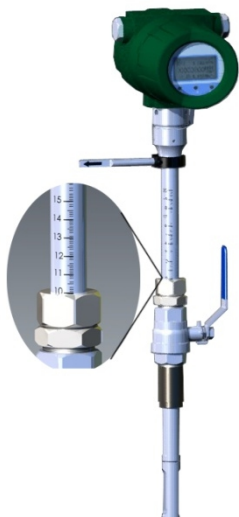
图 1 适用管径 DN100 以上 DN500 以下 精简型热式气体质量流量计
