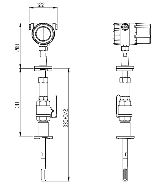
标准型外形尺寸
